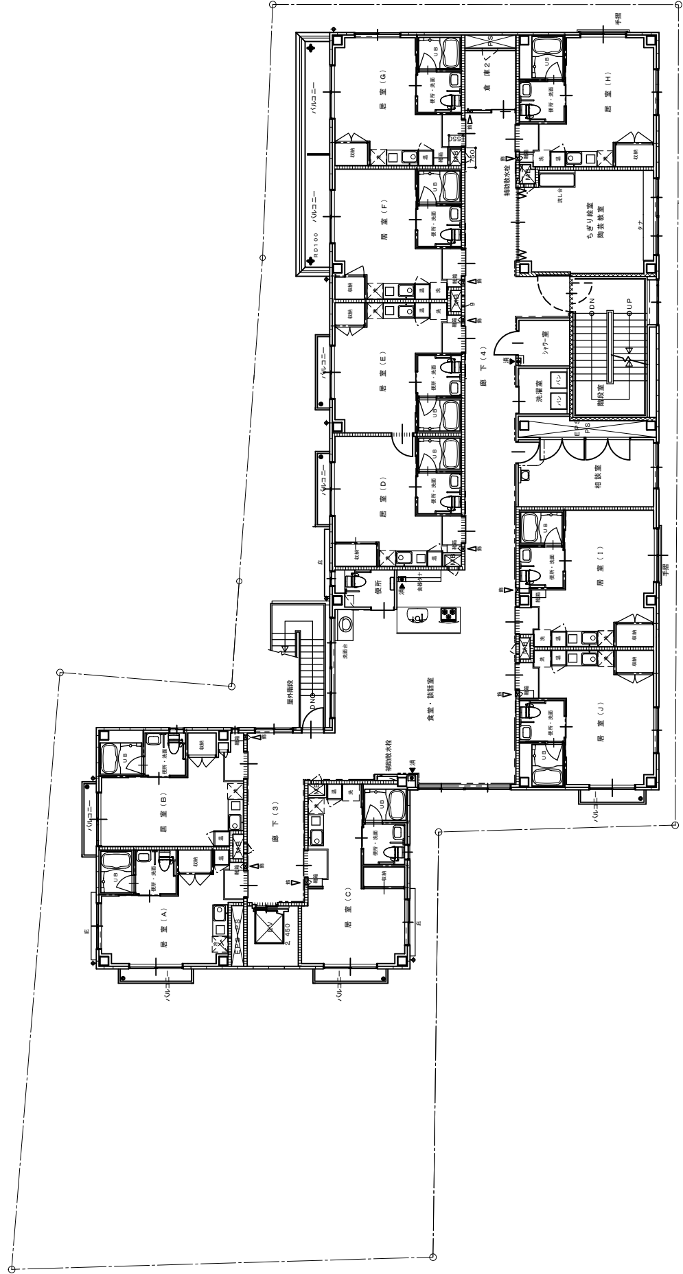
3 階 平 面 図 1 : 1 0 0
