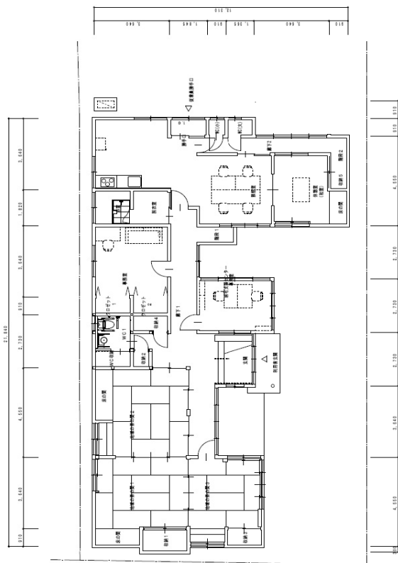
1階平面図
